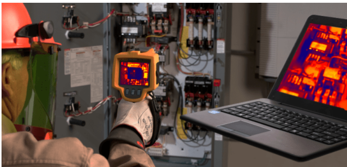
Рисунок 20. Пример проведения тепловизионного контроля электрошкафа
