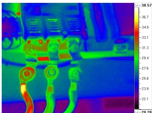
Рисунок 21. Пример термограммы контактных соединений с температурной шкалой
